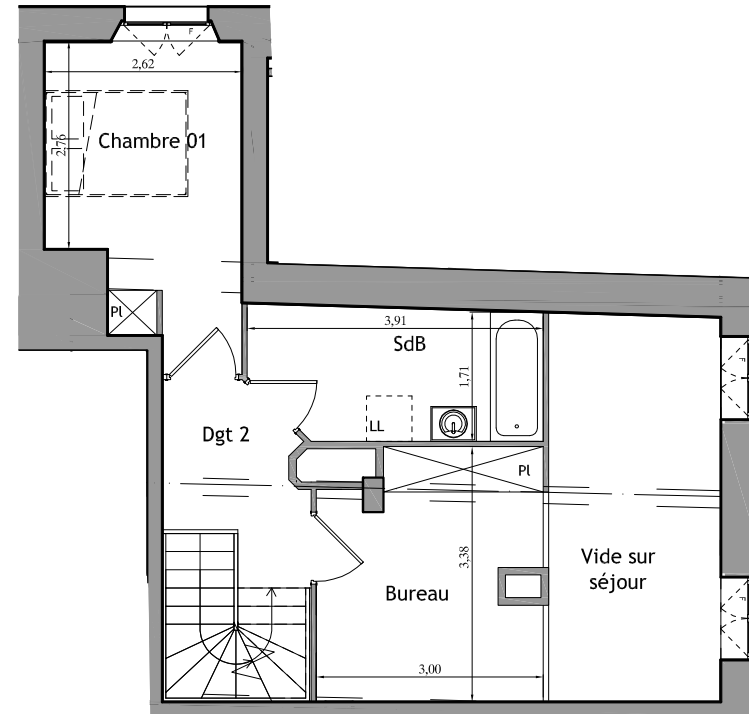
R+0,5 (hauteur sous plafond ≈ 2,20m)
